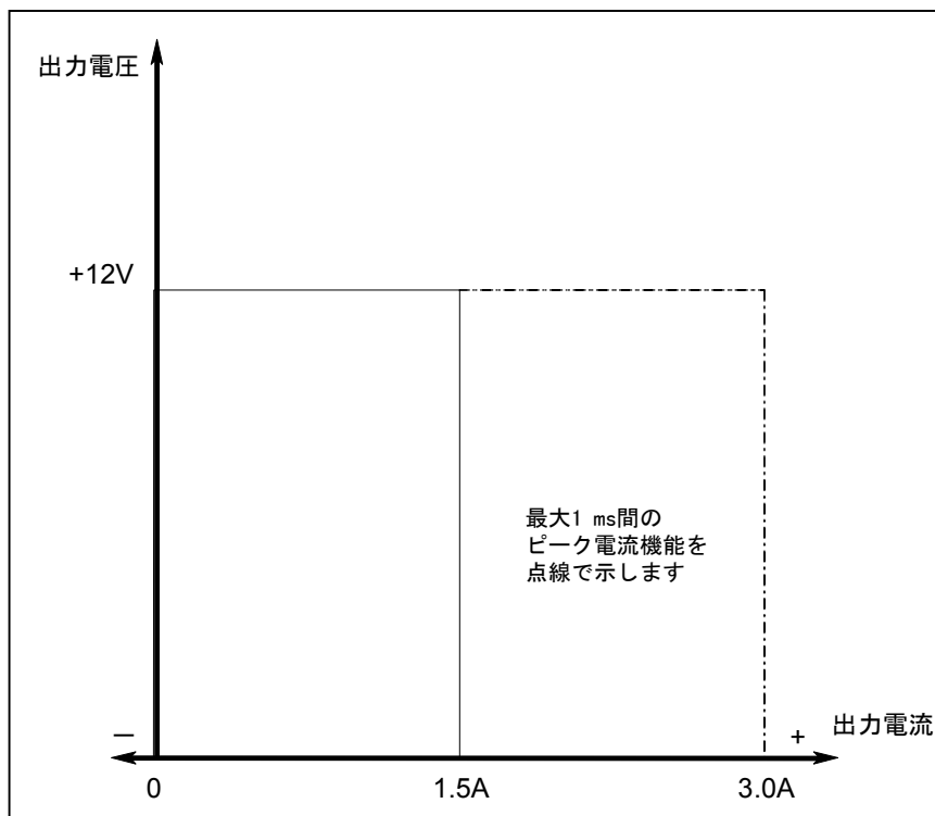
図 2-2. 出力2の特性
