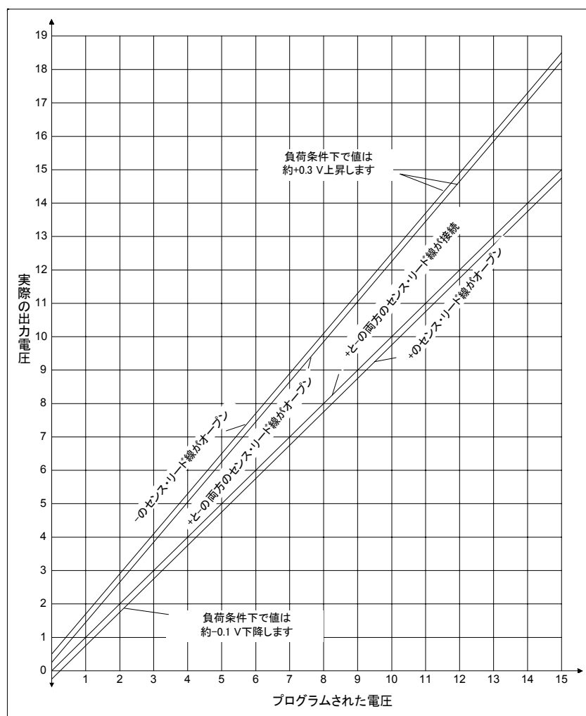
図 3-5. 出力電圧対オープン・センス条件でプログラムされた電圧
