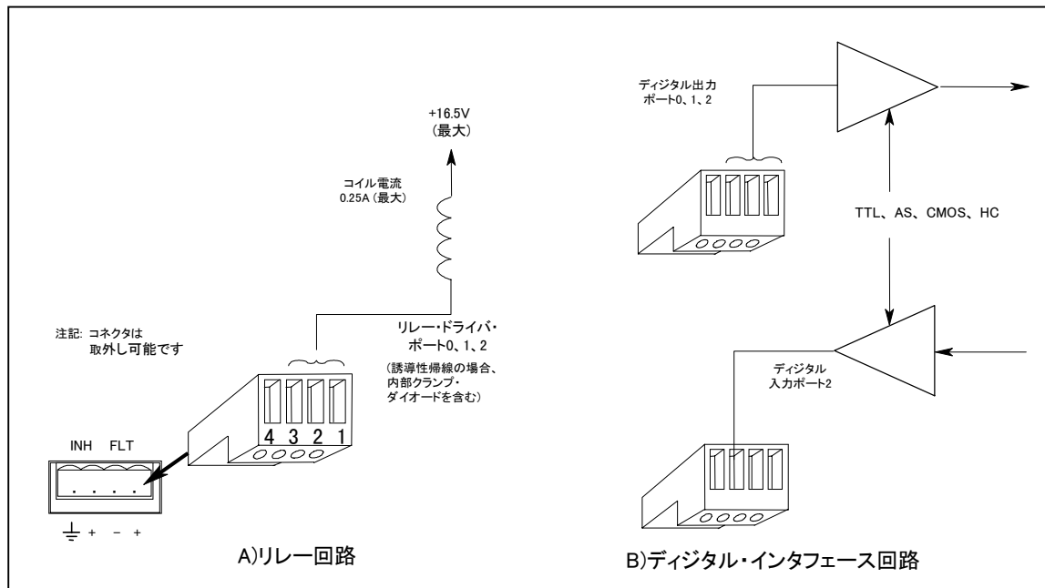
図 3-11. デジタルI/O例
