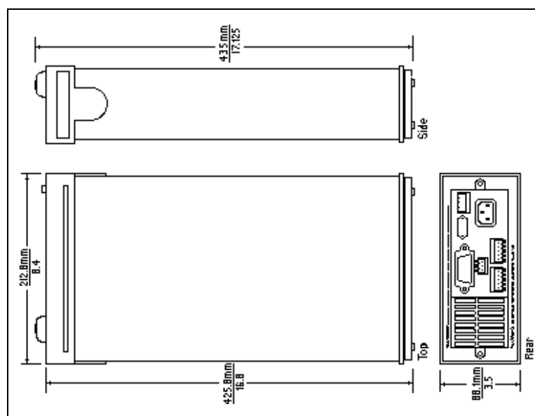
図 3-1. 外観図
