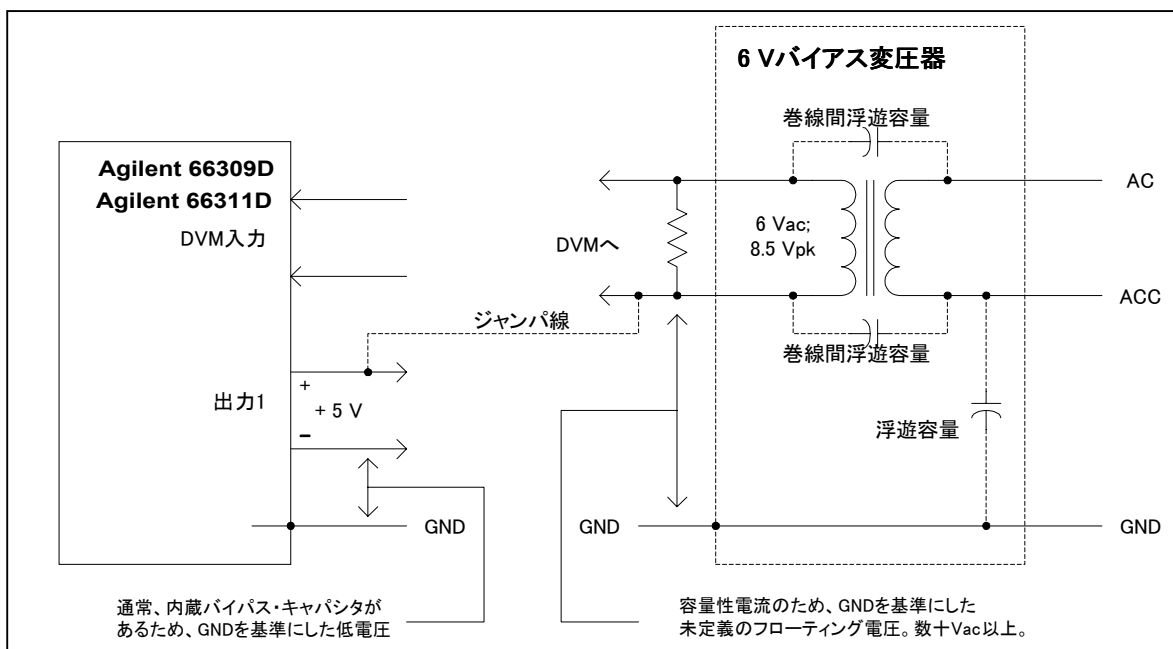
図 3-9. メイン出力を基準にしたフローティング回路の測定
