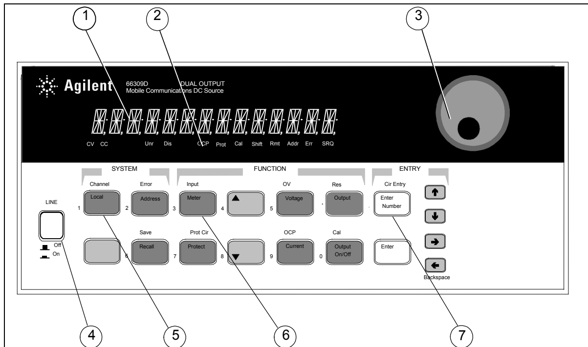
図 5-1. フロント・パネル全体図
