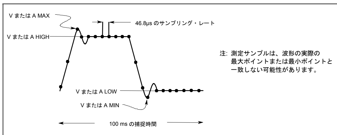
図 5-5. フロント・パネルのデフォルト測定パラメータ
