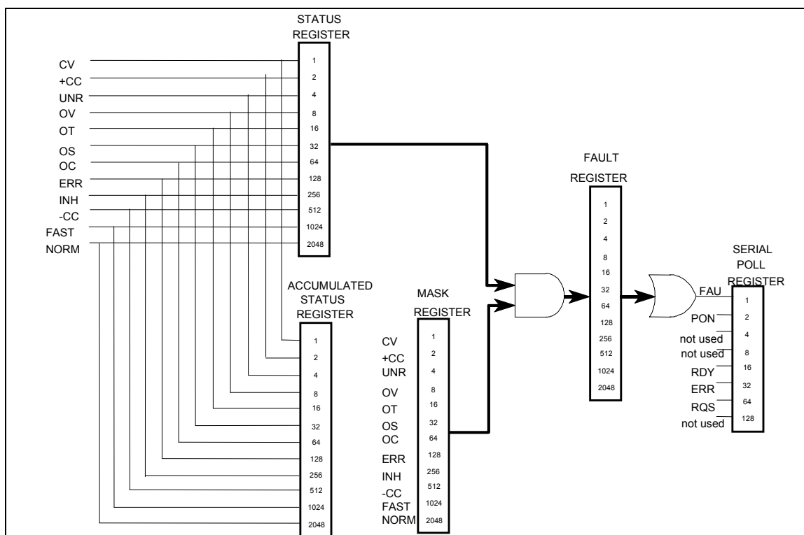
図 F-1. COMPatibilityステータス・モデル
