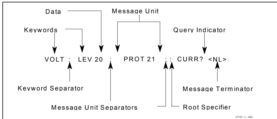
図 6-2 コマンド・メッセージの構造
