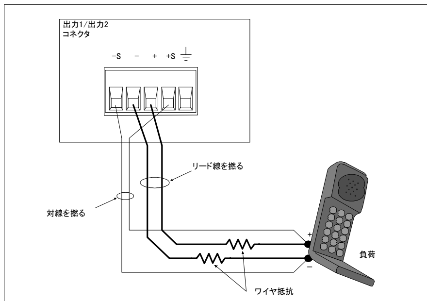
図 3-2. リモート・センス接続
