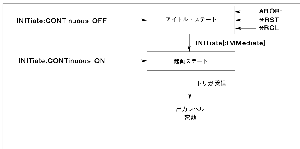
図 7-1 出力トリガのモデル
