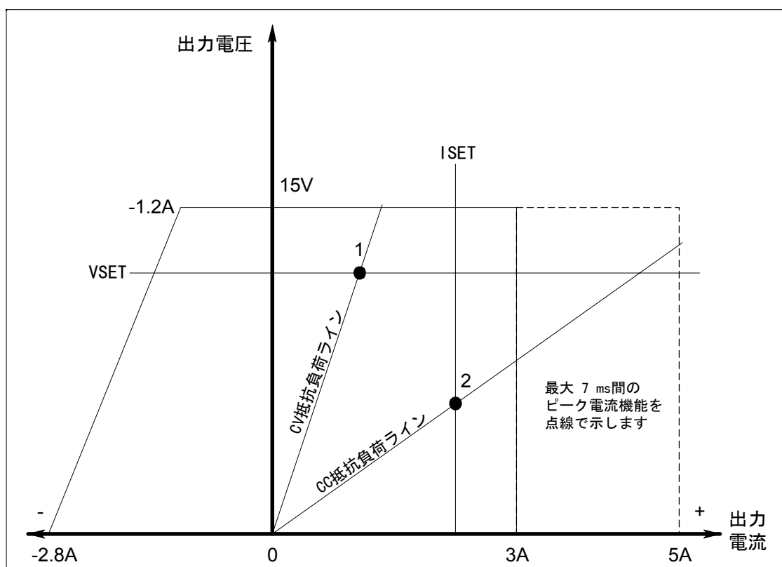
図 2-1. DCソース出力1の特性
