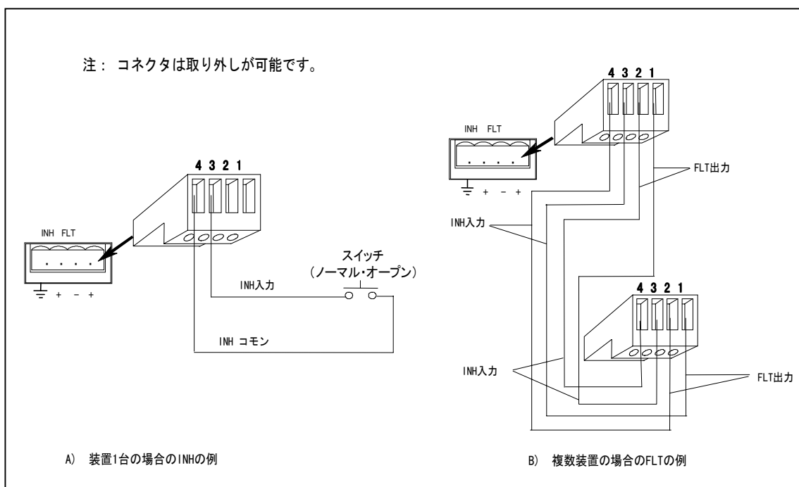
図 3-10. FLT/INHの例
