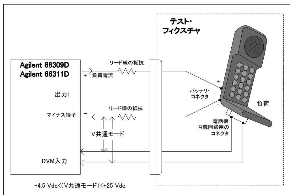
図 3-7. DVM測定の例
