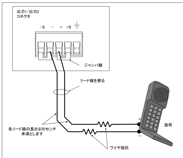
図 3-6. ローカル・センシング
